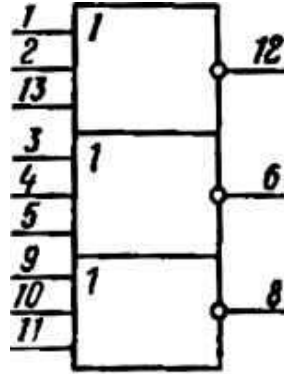
Условное графическое обозначение К555ЛЕ4, КМ555ЛЕ4
