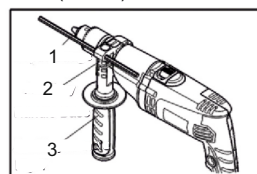
1.Глубиномер 2.Основание для вспомогательной ручки 3.Вспомогательная ручка
