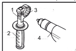
1.Основание для вспомогательной ручки 2.Вспомогательная ручка 3.Хомут 4.Углубление
