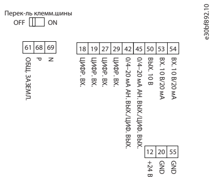
Рисунок 24: Клеммы управления
