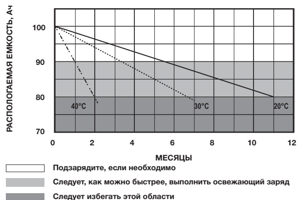
Рис. 8. Время хранения в зависимости от температуры воздуха
