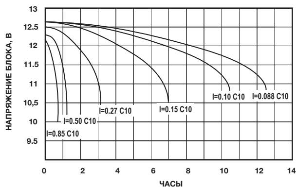
Рис. 1. Типичные кривые разряда для батарей AGM FIAMM (на примере батарей FIT)
