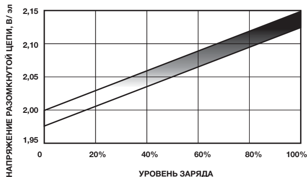
Рис.5 Приблизительный уровень заряда в зависимости от напряжения разомкнутой цепи AGM аккумулятора FIAMM
