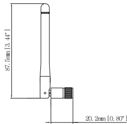
Antenna
