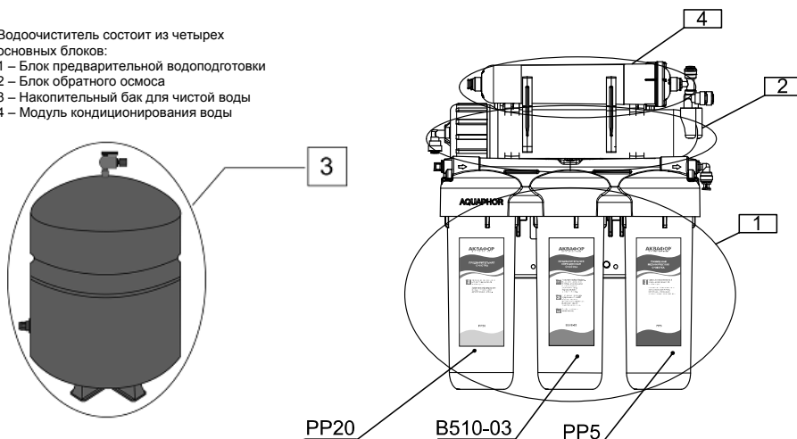
Рисунок 1. Блоки водоочистителя
