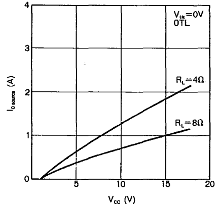
Fig. 6 出力ソース電流—電源電圧特性
