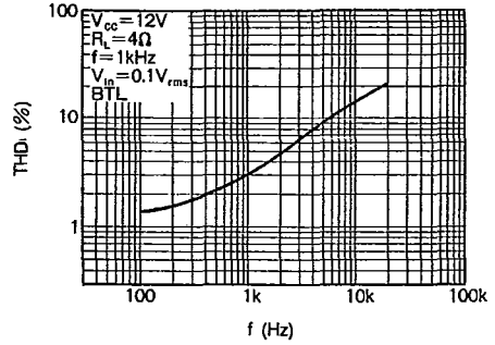
Fig. 4 歪率—周波数特性
