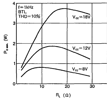
Fig. 8 最大出力電力—負荷抵抗特性
