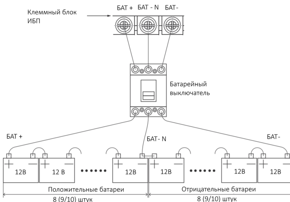
Рис. 3-4 Схема соединения на входе – «одна фаза + земля»
