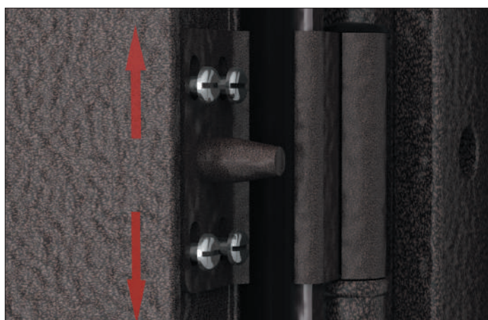
Двигая полотно двери вверх/вниз, выставите необходимый зазор и затяните винты крепления петель.
