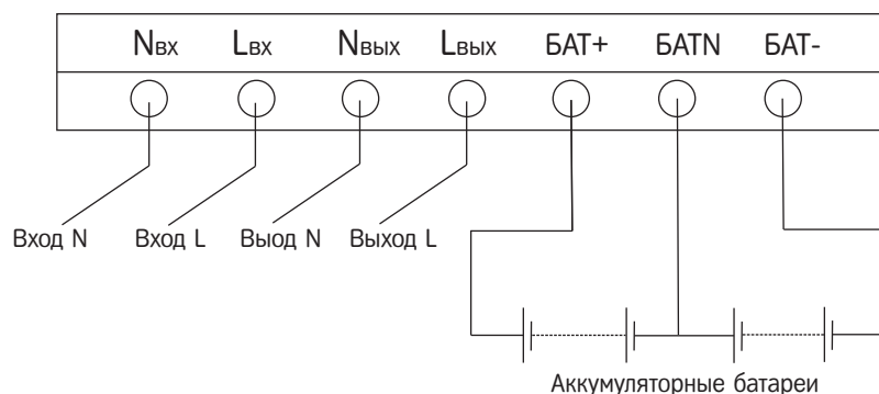
Рис. 3-4 Схема подключения входа и выхода ИБП
