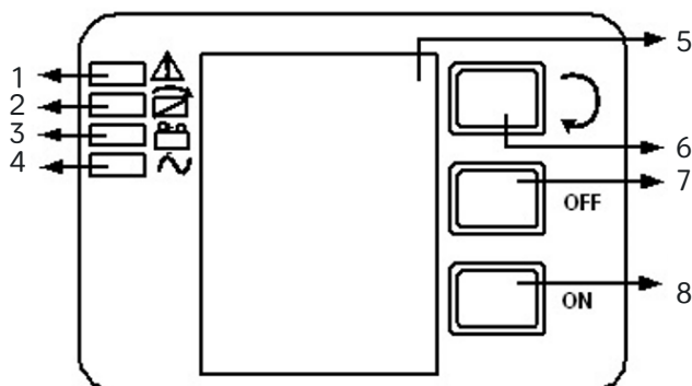
Рис. 3-2 Внешний вид панели управления
