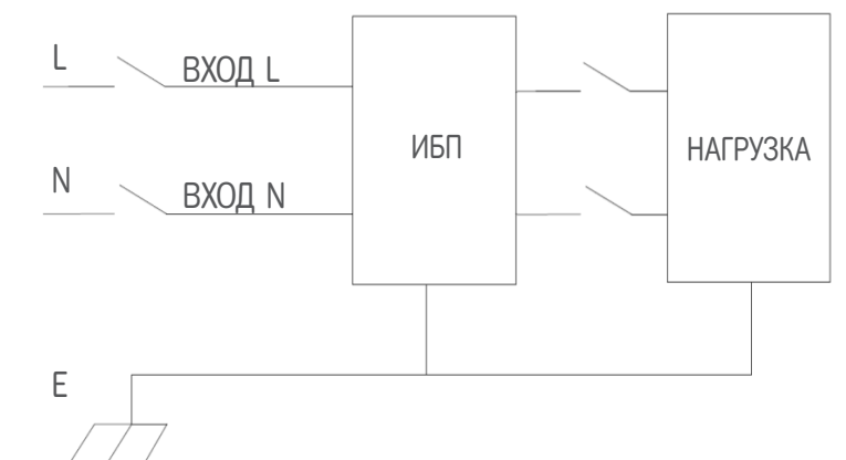
Рис. 3-3 Схема соединения на входе – «одна фаза + земля»
