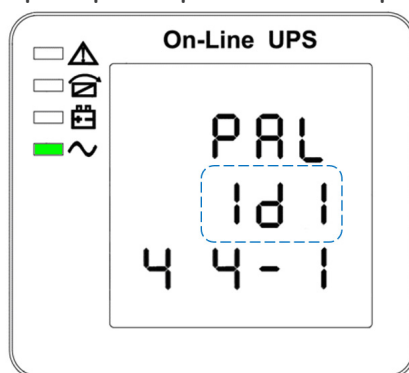
Рис. 4-12 Меню настройки идентификатора при параллельной работе ИБП (Примечание: изображение, выделенное пунктиром, мигает)
