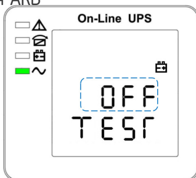
Рис. 4-11 Настройка тестирования АКБ
