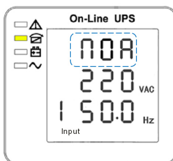
Рис. 4-3 Настройка режима работы
