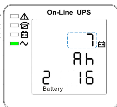
Рис. 4-6 Настройка ёмкости батареи (Примечание: изображение, выделенное пунктиром, мигает)
