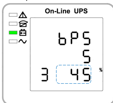
Рис. 4-9 Настройка параметров байпаса (Примечание: изображение, выделенное пунктиром, мигает)
