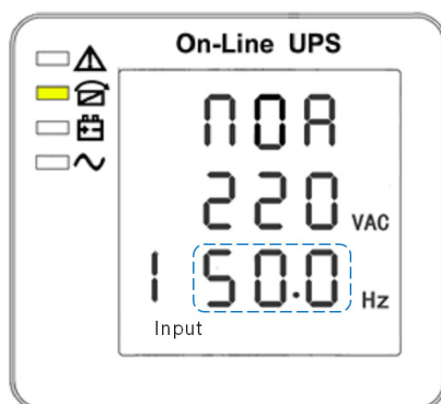
Рис. 4-5 Настройка выходной частоты (Примечание: изображение, выделенное пунктиром, мигает)
