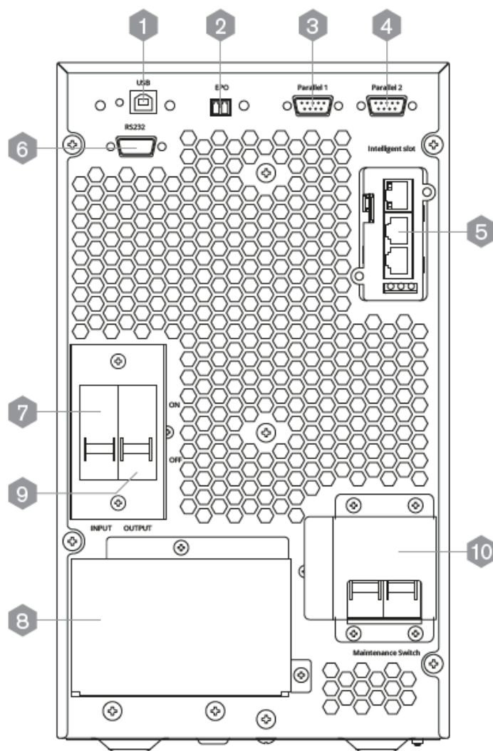
Рис. 3-1 Задняя панель
