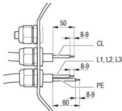
Иллюстрация 2: Рекомендованная длина зачистки концов кабеля, мм (внутри клеммной коробки)
