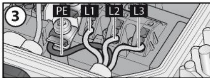
Иллюстрация 3: Подключение проводов к клеммам ⇒ Уплотните клеммную коробку.
