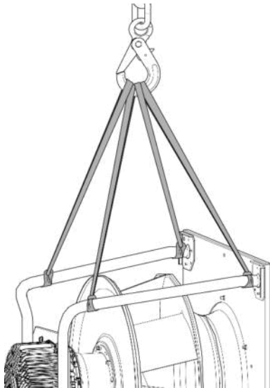
Иллюстрация 1: Схема подъема для транспортировки RadiPac
