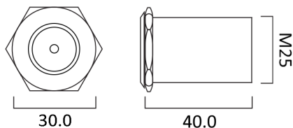
Рис.1 Считыватель QR-X-2 (врезной). Габариты изделия.
