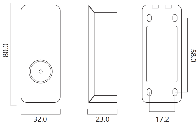
Рис.2 Считыватель QR-X-3 (накладной). Габариты изделия.
