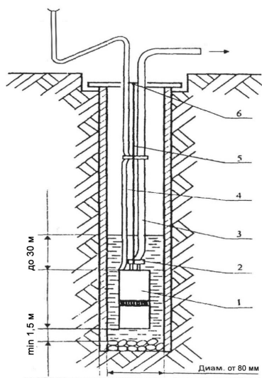
Рис. 3 Схема установки электронасоса Belamos TS в скважину 1 – электронасос; 2 – хомут шланга; 3 – шланг; 4 – электрокабель; 5 – трос; 6 – место крепления подвески.
