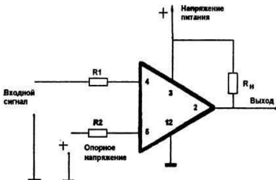
Схема включения одного канала К1401СА2; R_1 = R_2 = 0 \dots 10 \text{ кОм}
