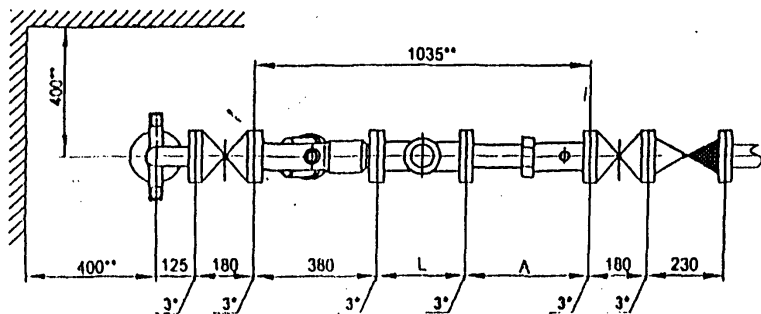
Установка счетчика d_u=50 мм (турбинного) с с фильтром-струвыпрямителем (ФС) в водомерном узле на вводе диаметром 50 мм. Схема водомерного узла.
