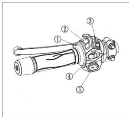
Рис. 8 Левый блок управления
