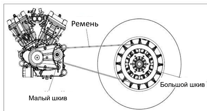
Рис. 21 Ременный привод
