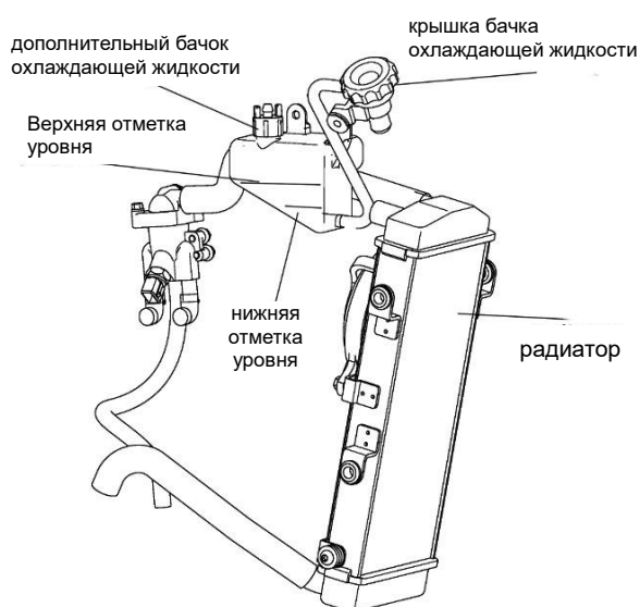
Рис. 32 Система охлаждения
