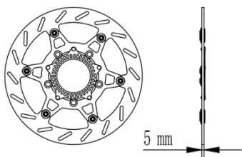
Рис.25. Проверка переднего тормозного диска
