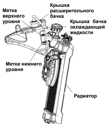
Рис. 33. Система охлаждения
