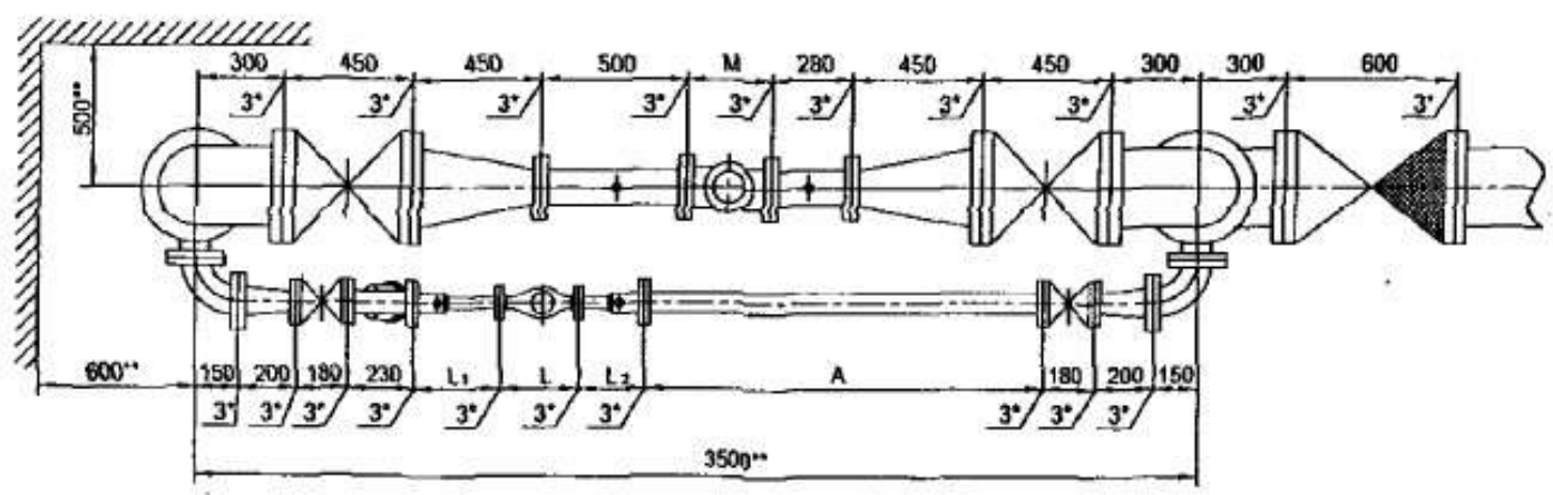
Установка счетчиков du=20 \dots 50 мм на хозяйственно-питьевой линии и счетчика du=100 мм на пожарно-резервной линии в водомерном узле на вводе диаметром 250 мм. Схема водомерного узла.
