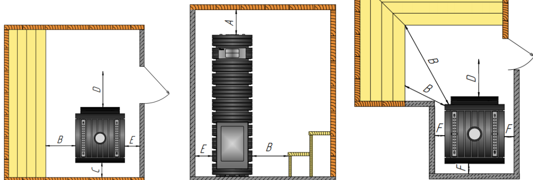
Рисунок 4. Безопасные расстояния
