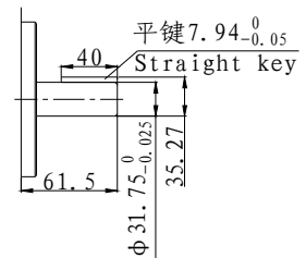
2号轴 (NO SAE) No2. Shaft
