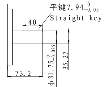
2号轴 (NO SAE) No2. Shaft
