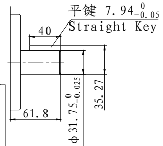
2号轴 (NO SAE) NO. 2 Shaft
