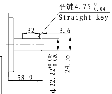
2号轴 (NO SAE) No2. Shaft
