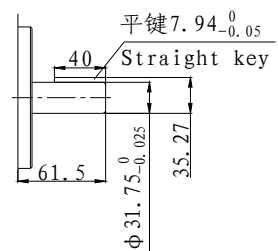
2号轴 (NO SAE) No2. Shaft
