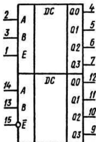
Условное графическое обозначение КР1561ИД7
