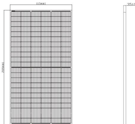
а) Вид спереди б) Вид сбоку Рисунок 1 – Схематическое изображение ФЭМ.
