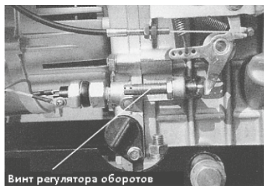
Рис. 7. Регулятор оборотов
