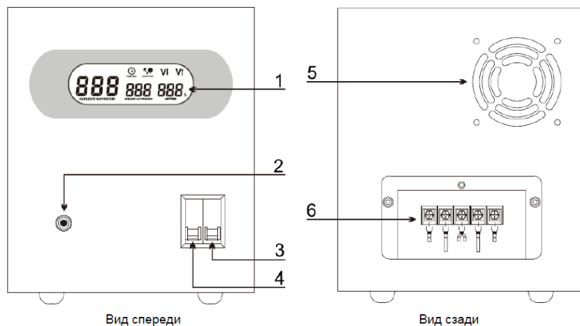
Рисунок 1. Внешний вид стабилизаторов напряжения SMARTWATT AVR STRONG 15000-20000VA. Описание элементов приводится в таблице 1.
