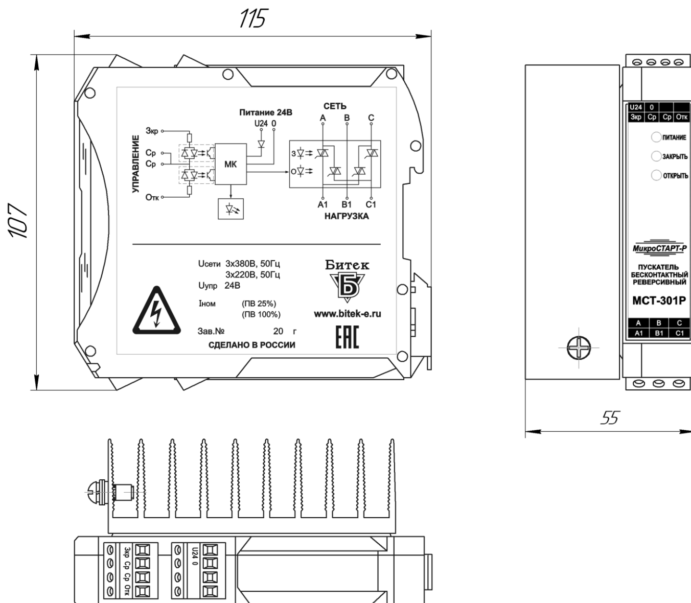
Рисунок А.2 – Габаритно-установочные размеры МСТ-301Р
