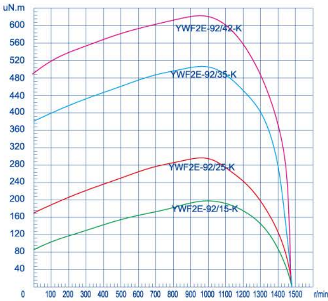
Torque(50Hz)
