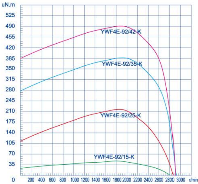
Torque(50Hz)
