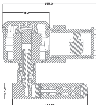
Секция А - А
