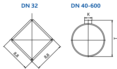
Размеры штока
