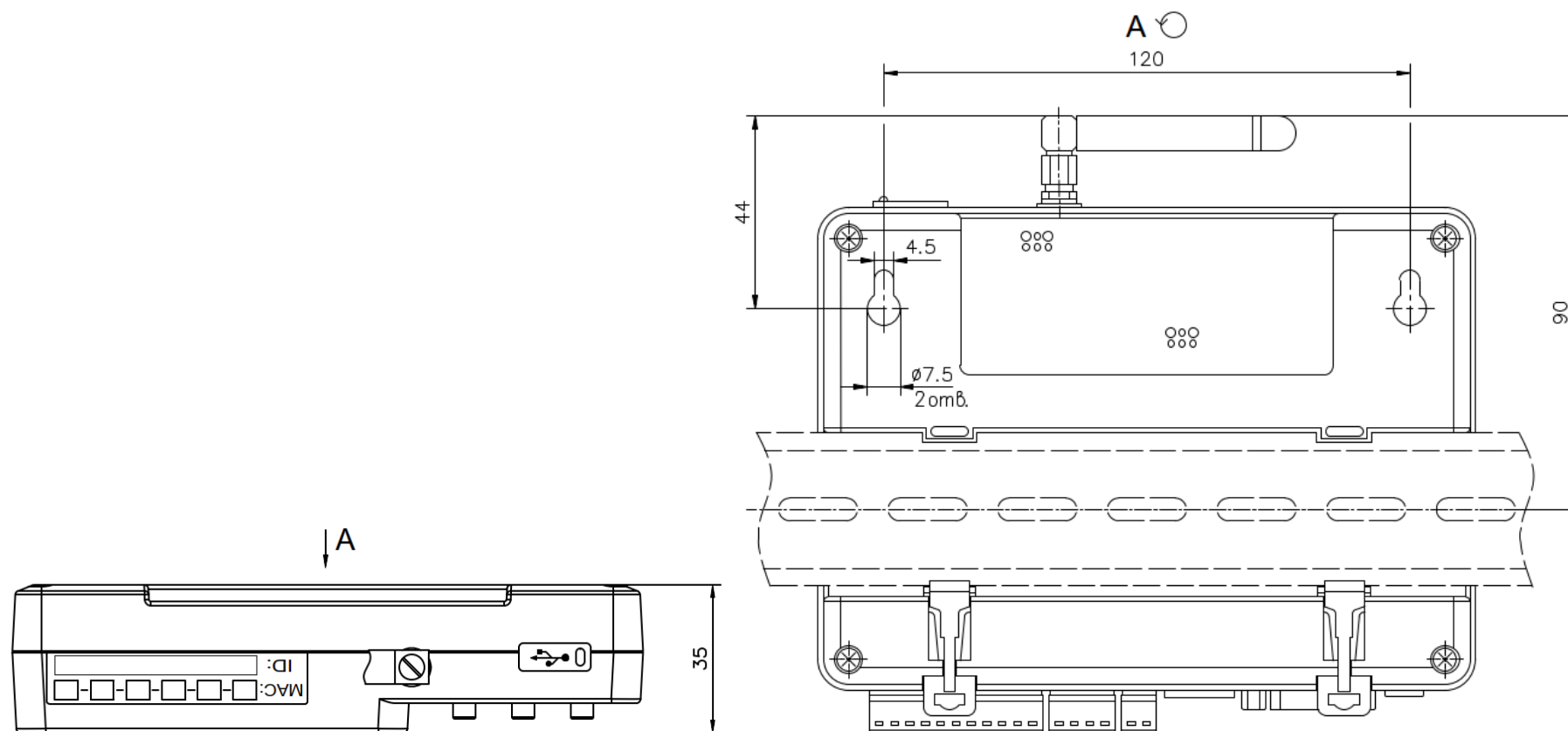
Рисунок А.3 – Габаритные размеры ЛБ7.3 (с DIN-рейкой)
