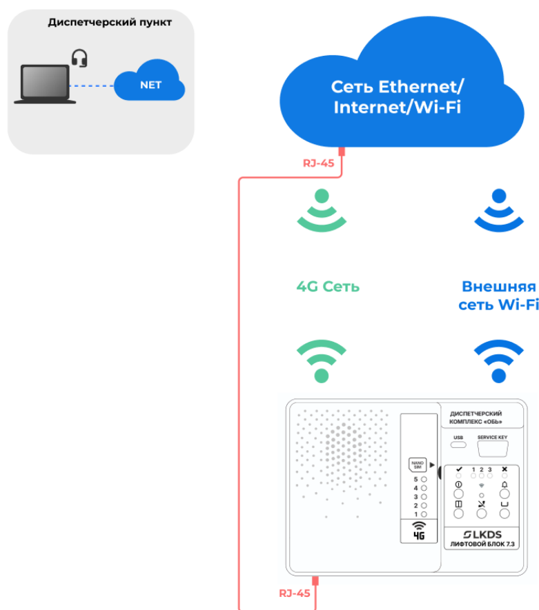
Рисунок 5 – Подключение лифтового блока 7.3 к внешней сети передачи данных
