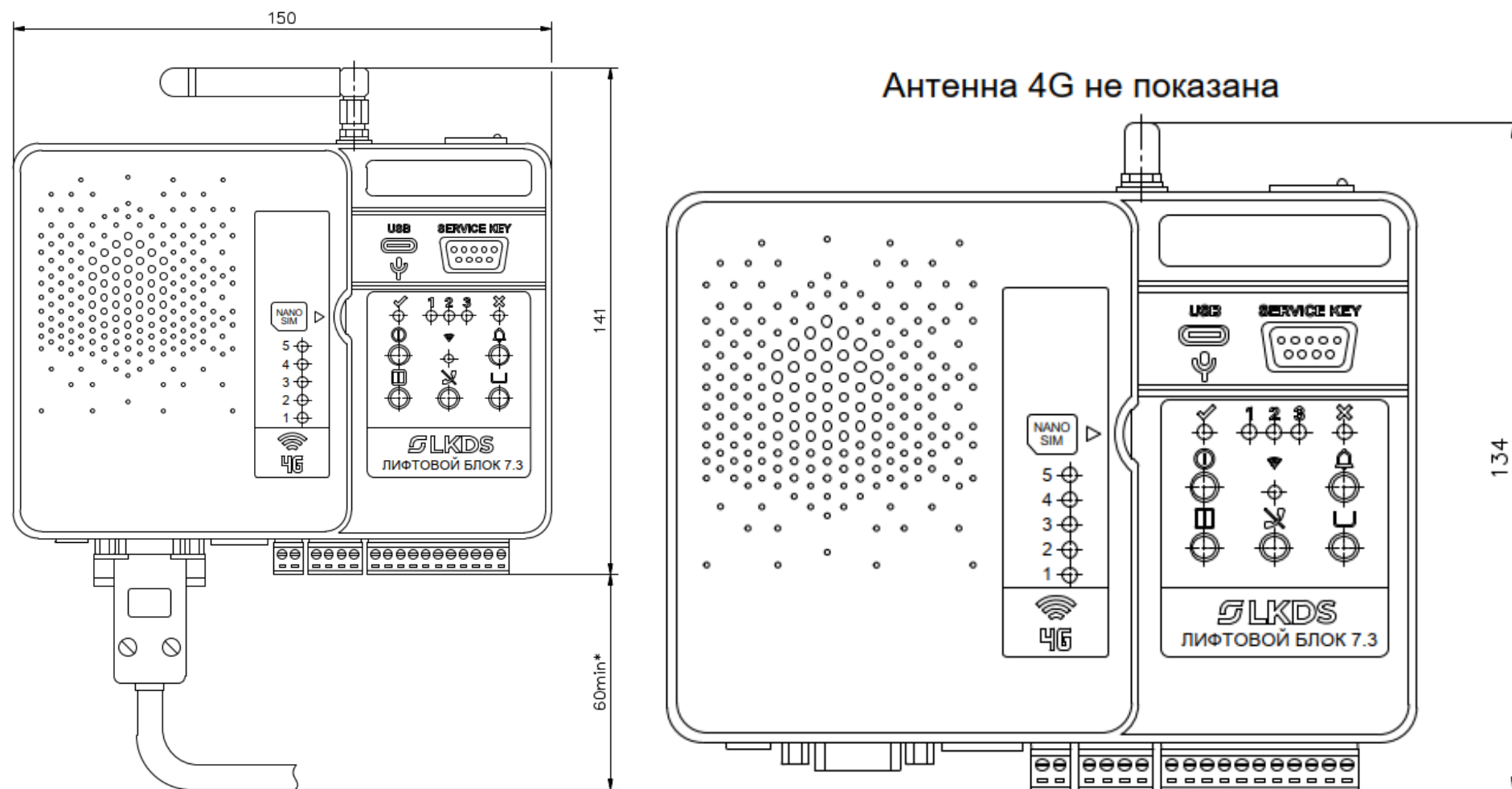
Рисунок А.1 – Габаритные размеры ЛБ7.3
