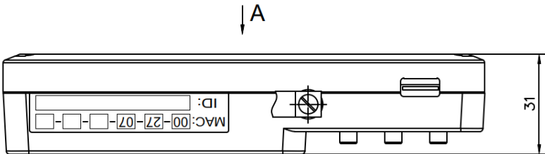
Рисунок А.2 – Габаритные размеры ЛБ7.3 (без DIN-рейки)
