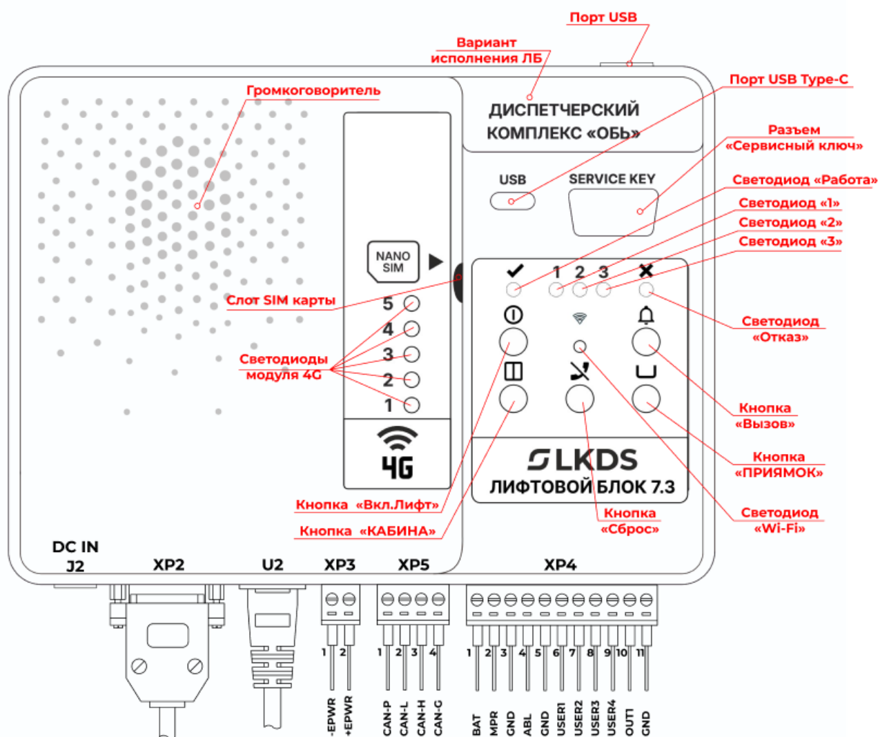
Рисунок 1 – Внешний вид лифтового блока 7.3, назначение разъемов, органов управления и индикации
