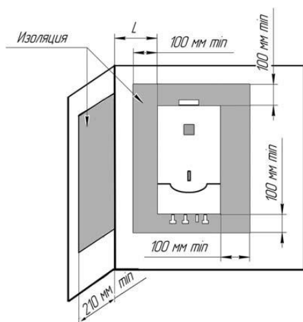
Рис. Установка аппарата на трудносгораемых стенах.
