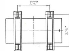
Колея для поперечного перемещения
