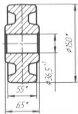
Каток (12,5)
