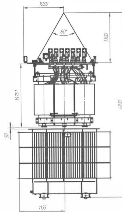
Подъем активной части
