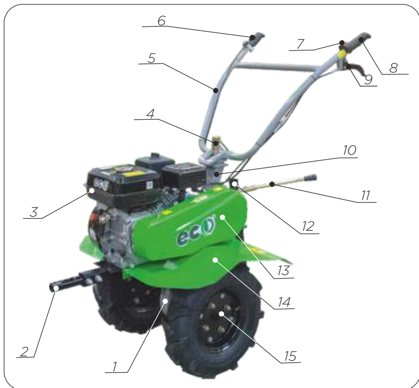
Рис.1 Мотоблок (общий вид)
