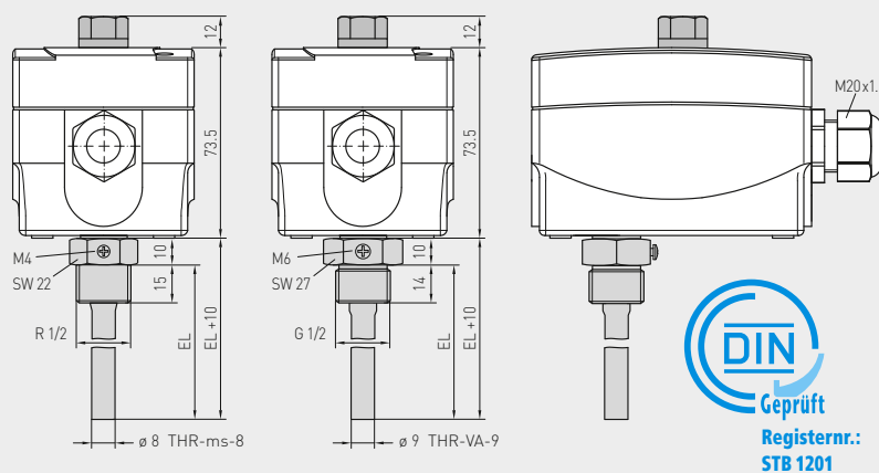
Габаритный чертеж регулируемый предохранительный ограничитель температуры STB
