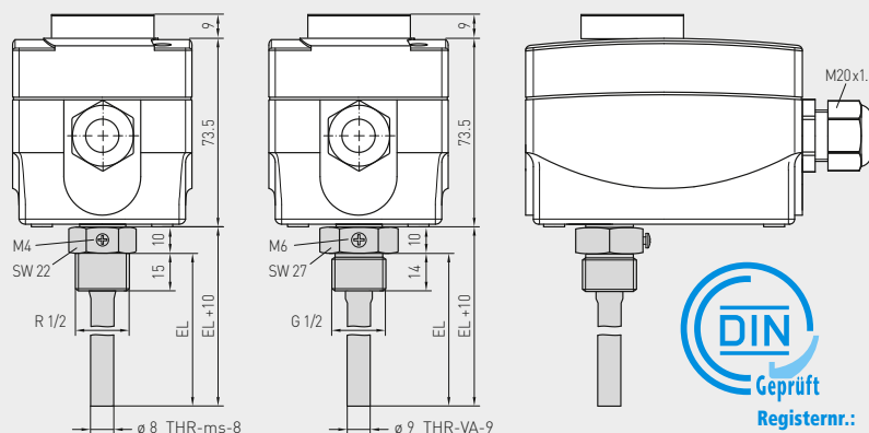
Габаритный чертеж Терморегулятор TR
