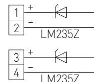
1 двухпроводное отключение LM 235 Z (KP 10)
