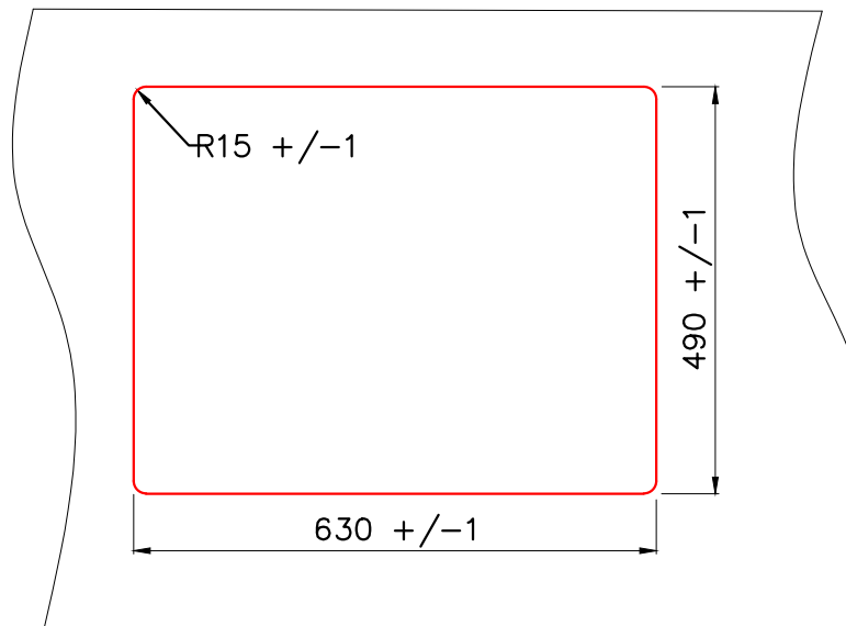
Врезной монтаж мойки (I)
