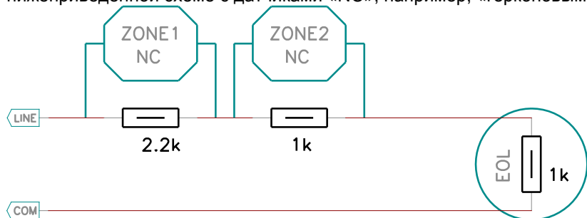
Рис. 24 Пример подключения двух герконовых датчиков (из стандартного комплекта Устройства)
