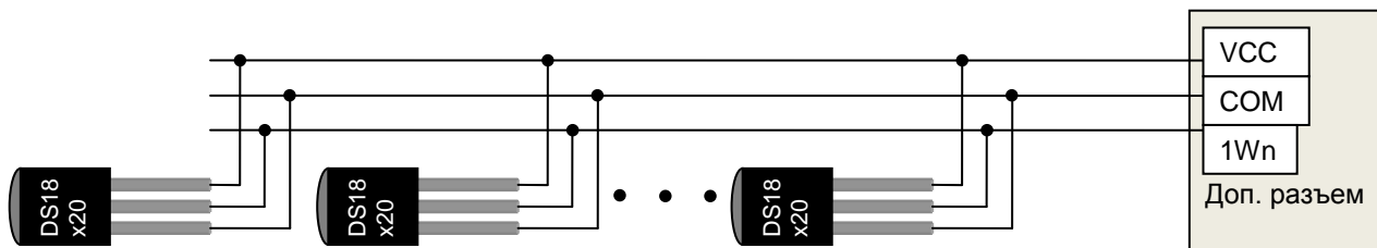
Рис. 16 Способ подключения датчиков DS18S20/DS18B20 по 3-проводной шине
