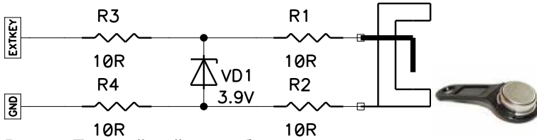
Рис. 17 Простейший способ защитить входную цепь от применения высоковольтного «шокера»
