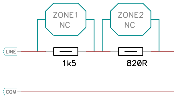
Рис. 27 Пример подключения двух герконовых датчиков (из стандартного комплекта Устройства)
