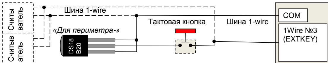
Рис. 18 Способ подключения считывателя IButton и кнопки установки на «охрану периметра»
