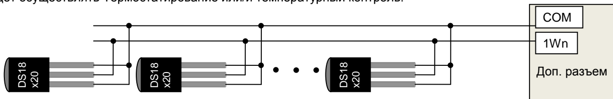
Рис. 15 Способ подключения датчиков DS18S20/DS18B20 по 2-проводной шине
