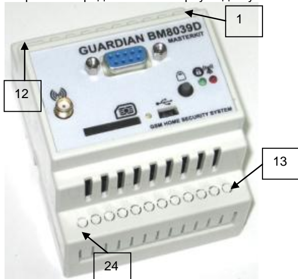
Рис. 5 Внешний вид блока
