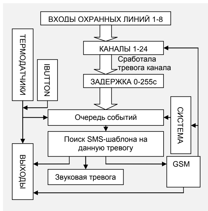
Рис. 1 Алгоритм работы устройства
