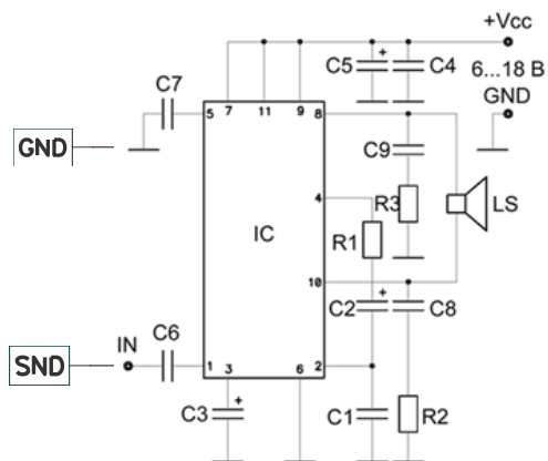
Рис. 20 Пример подключения сирены через усилитель ВМ057
