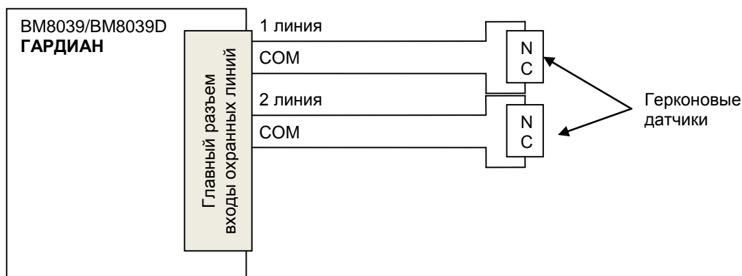
Рис. 23 Пример подключения двух герконовых датчиков (из стандартного комплекта Устройства)
