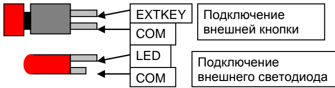
Рис. 12 Подключение элементов управления
