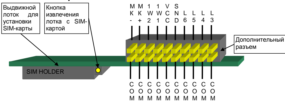
Рис. 10 Вид платы со стороны дополнительного разъема
