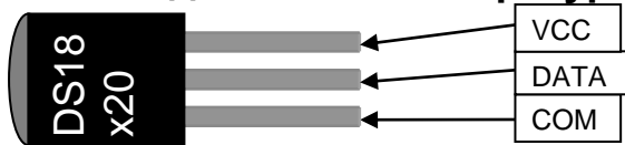
Рис. 14 Распиновка датчика температуры DS18B20/DS18S20/DS1822
