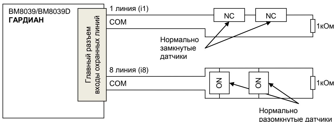
Рис. 22 Пример подключения нормально разомкнутых и нормально замкнутых датчиков в режиме контроля сопротивления линии
