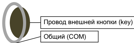
Рис. 2 Подключение считывателя IButton (схематическое изображение)
