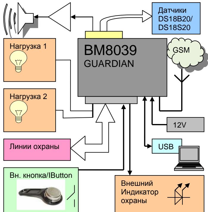
Рис. 4 Схема подключения устройства
