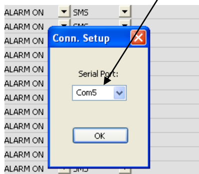
Рис. 29 Установка соединения
