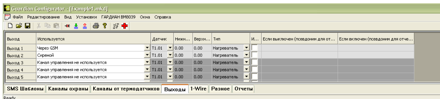
Рис. 35 Настройка выходов
