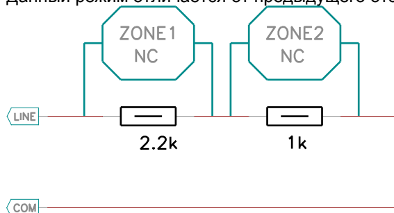
Рис. 25 Пример подключения двух герконовых датчиков (из стандартного комплекта Устройства)
