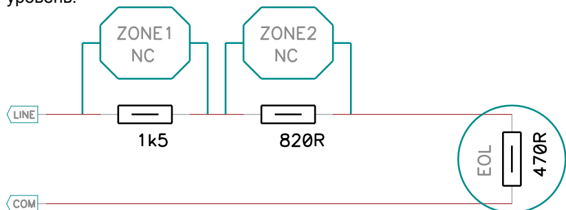
Рис. 26 Пример подключения двух герконовых датчиков (из стандартного комплекта Устройства)
