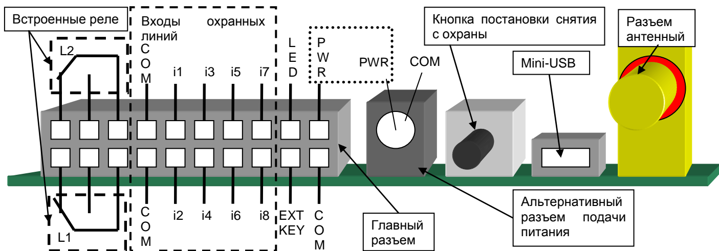
Рис. 9 Вид платы со стороны главного разъема
