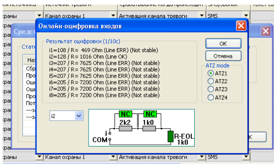
Рис. 43 Онлайн-оцифровка входов
