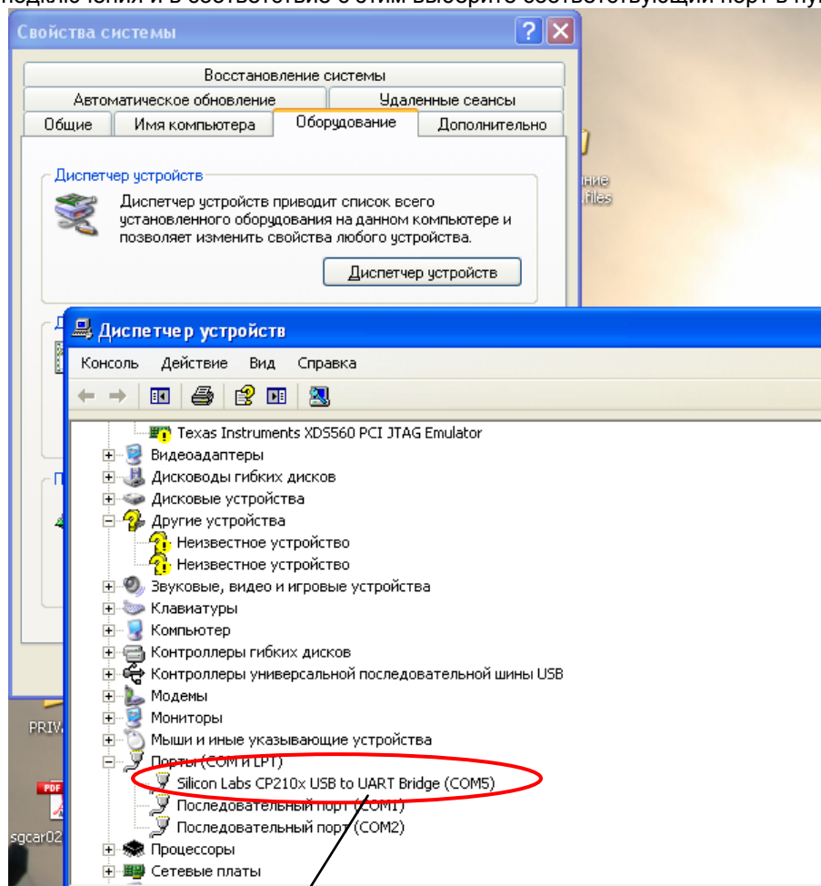
Рис. 28 Диспетчер устройств
