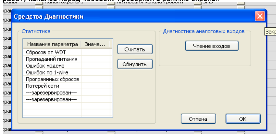
Рис. 42 Средства диагностики
