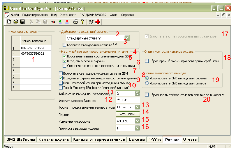
Рис. 38 Разное
