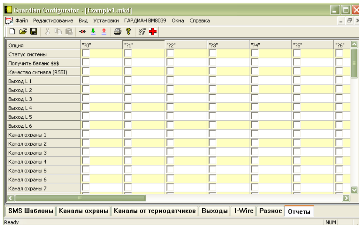
Рис. 39 Отчеты
