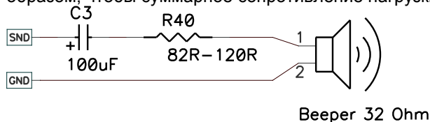
Рис. 21 Пример подключения динамика напрямую к охранному блоку
