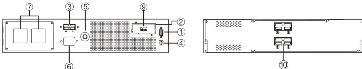
Monolith V 1000RT(LT)/2000RT(LT)/3000RT(LT) и батарейный блок
