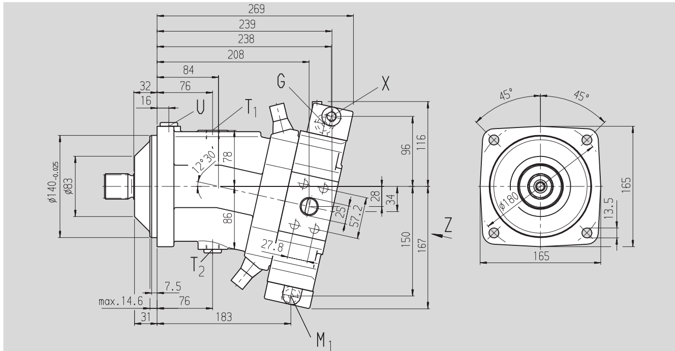
Вид Z Рабочие присоединения A/B сбоку, противоположно (02) Рабочие присоединения A/B сзади (01)
