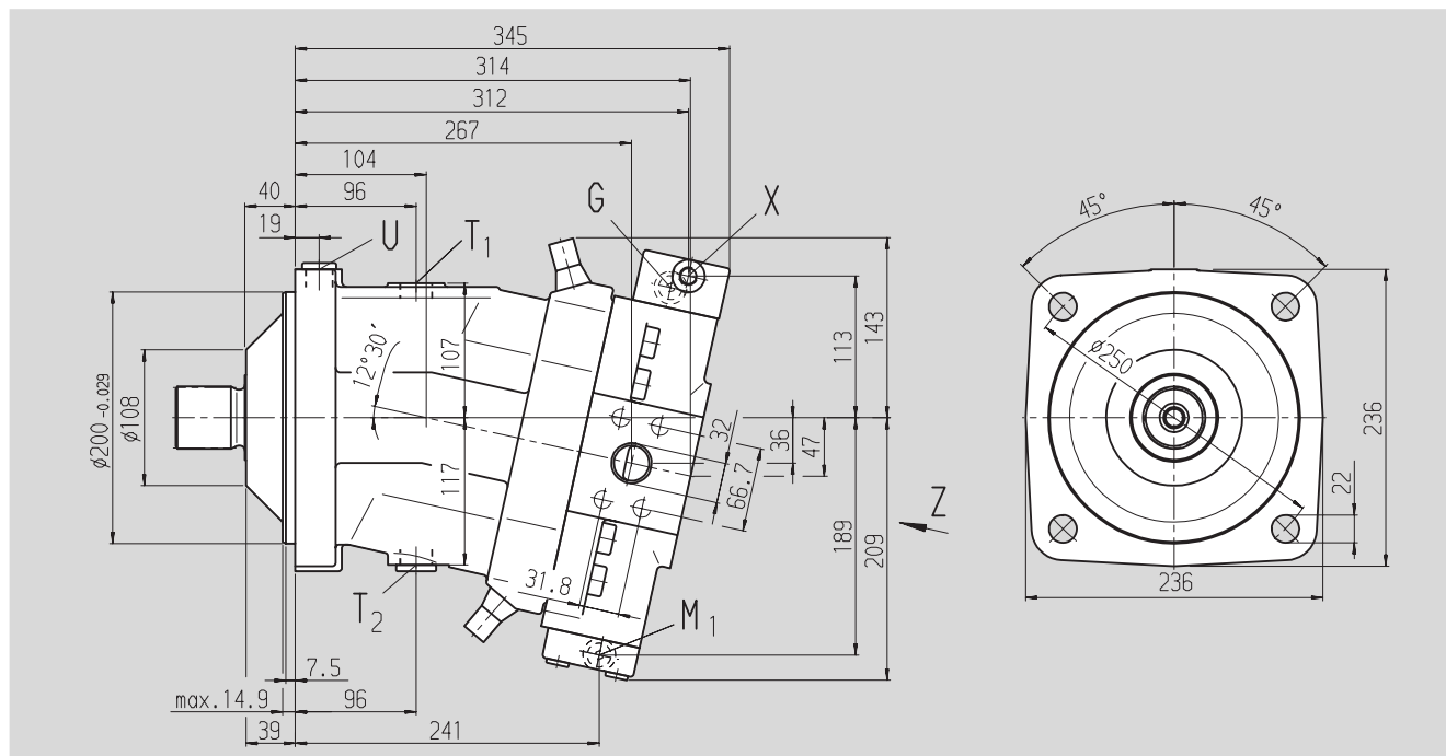
Вид Z
