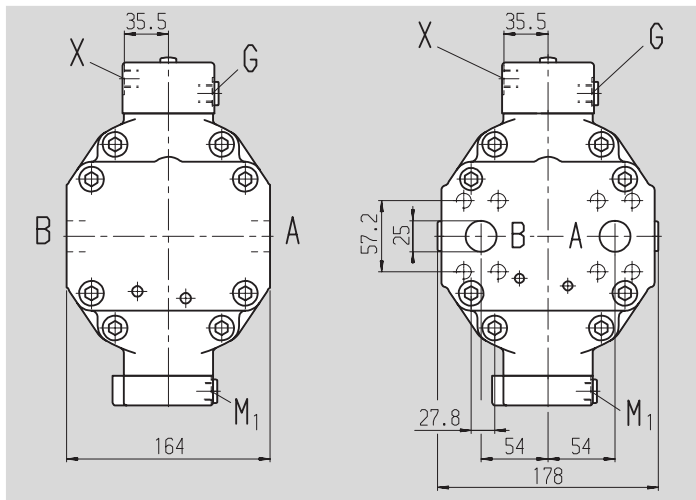
Вид Z Рабочие присоединения A/B сбоку, противоположно (02) Рабочие присоединения A/B сзади (01)
