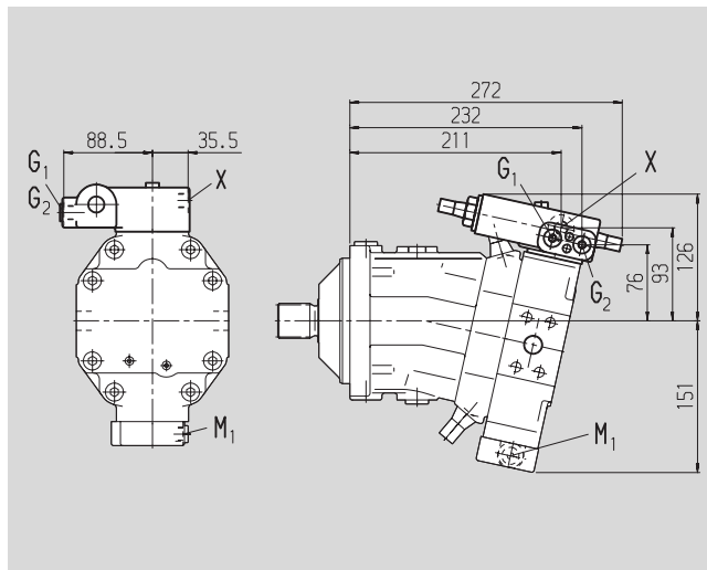
Электрическое управление с пропорциональным магнитом, EP1, EP2
