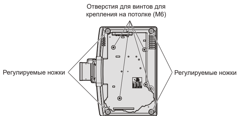
Положения отверстий для винтов для крепления на потолке и регулируемых ножек
