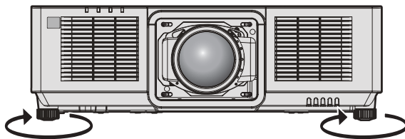
Максимальный диапазон настройки Регулируемые ножки: 23 мм (29/32") каждая
