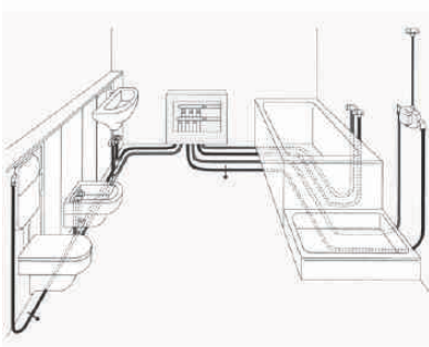
Рисунок 31. Пример разводки с применением коллекторов. Royal Thermo.
