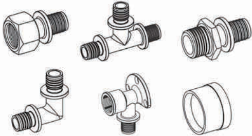
Рисунок 4. Фитинги AXIOpress
