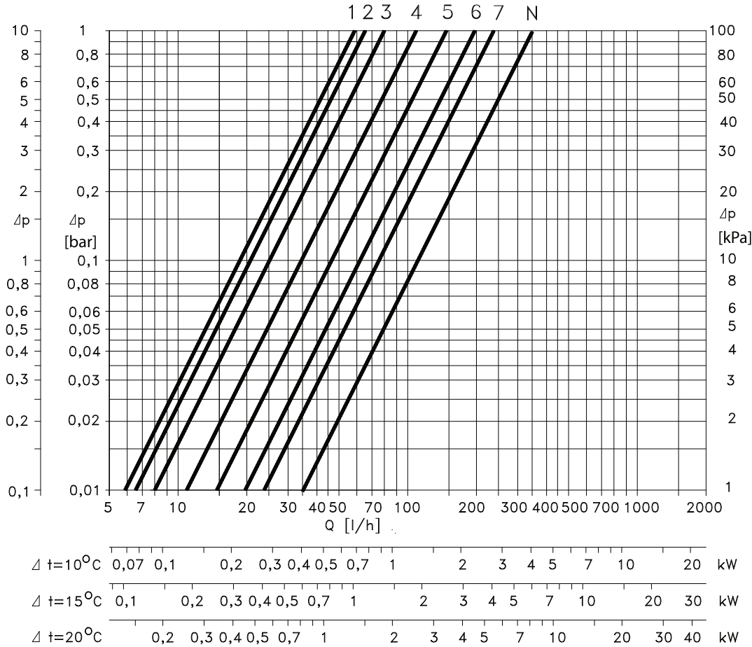
Диаграмма для определения предварительной настройки клапана RA-U 013G1383 с установленным термоэлементом серии RA 2000 при \chi_p=2^{\circ}\text{C}
