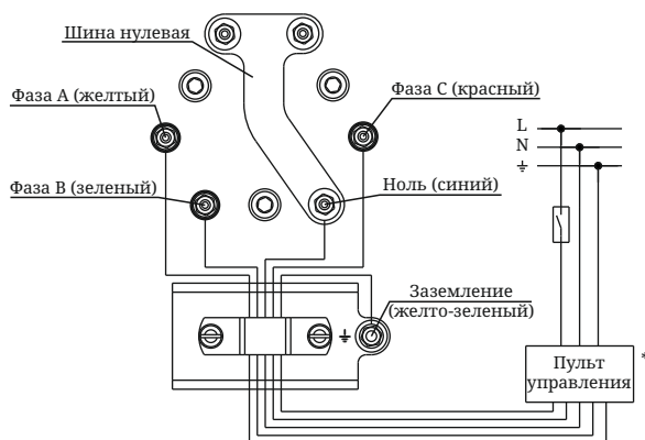
Рисунок 6. Монтажная схема подключения электрокаменки к однофазной сети
