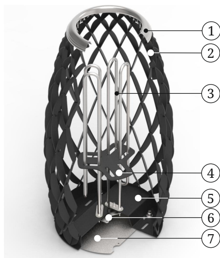
Рисунок 2. Расположение основных элементов электрокаменки «Мэри Экс».
