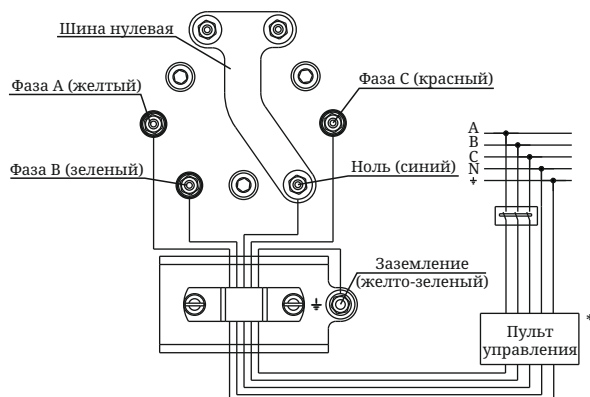
Рисунок 5. Монтажная схема подключения электрокаменки к трехфазной сети
