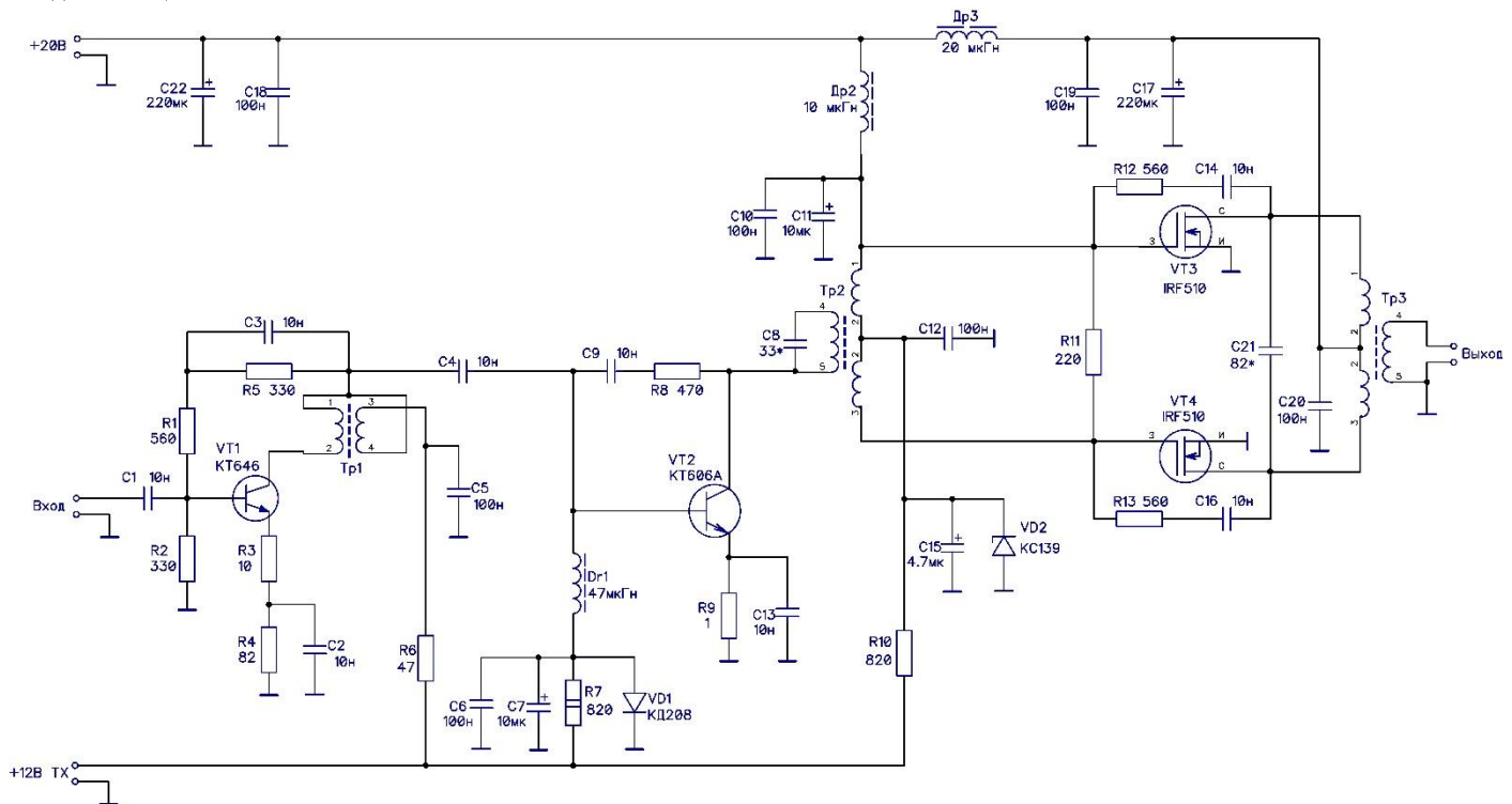
Принципиальная схема усилителя мощности "Дружба". Плата UM-U-IRF. Версия платы 2.0
