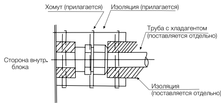
Изоляция труб
