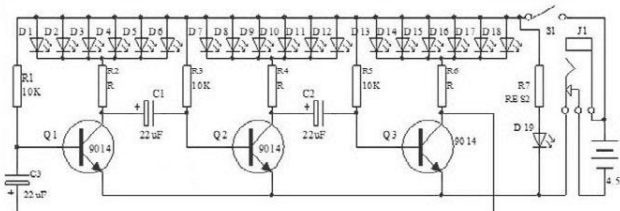
Монтажная схема платы SH-C
