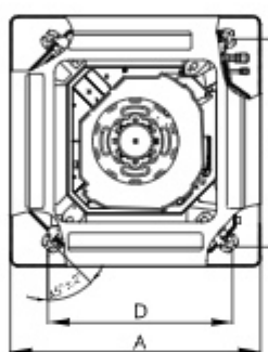
Внешние размеры панели
