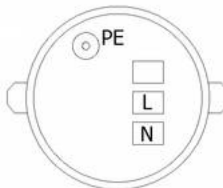
Рисунок 2 – Подключение
