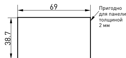
Установка винтов: чертеж с размерами прорези в панели
