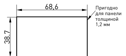
Установка винтов: чертеж с размерами прорези в панели
