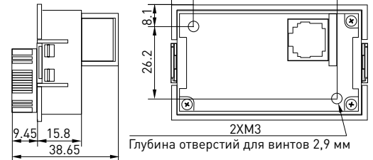
Установочные размеры выносного пульта управления DU06
