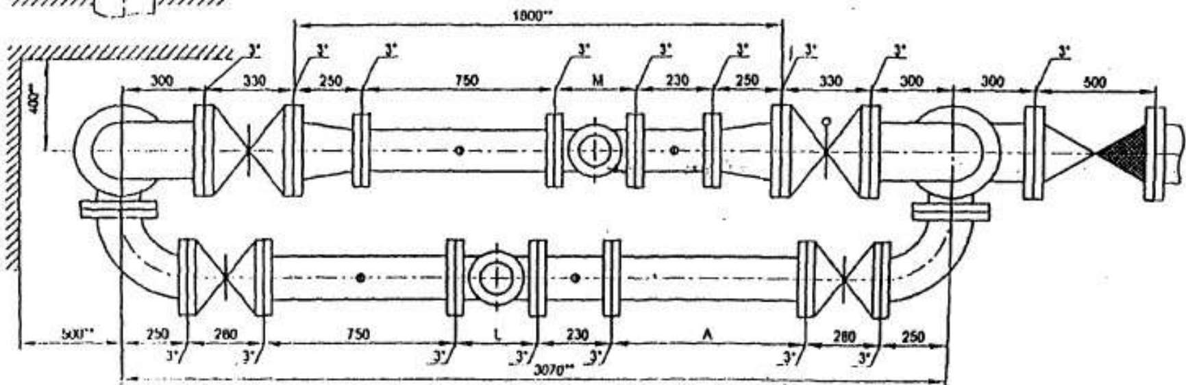
Установка счетчика d_u=150 мм на хозяйственно-питьевой линии и счетчика d_u=150 мм на пожарно-резервной линии в водометном узле на входе диаметром 200 мм. Схема водометного узла.
