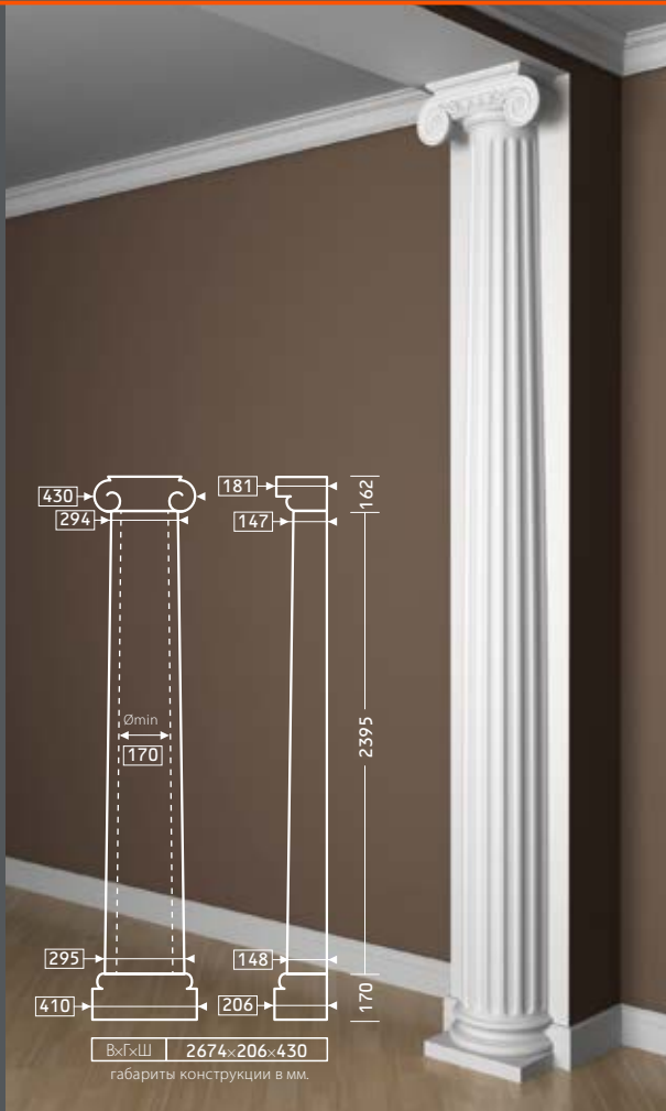
КАПИТЕЛЬ 4.15.201 СТВОЛ 4.16.201
