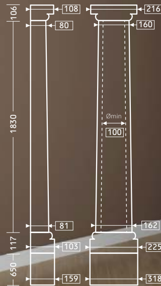
БАЗА 1.17.700
