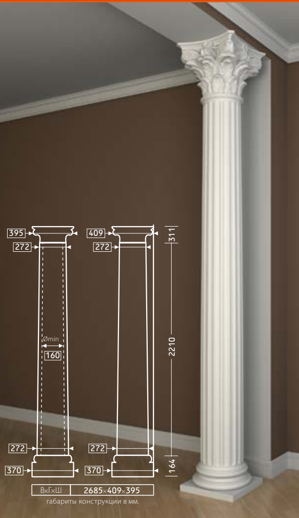
СТВОЛ 4.12.301
