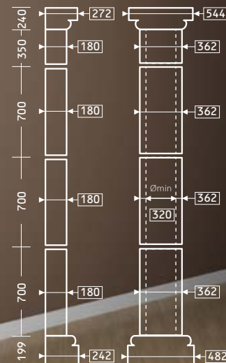
БАЗА 4.17.001 СТВОЛ 4.16.002
