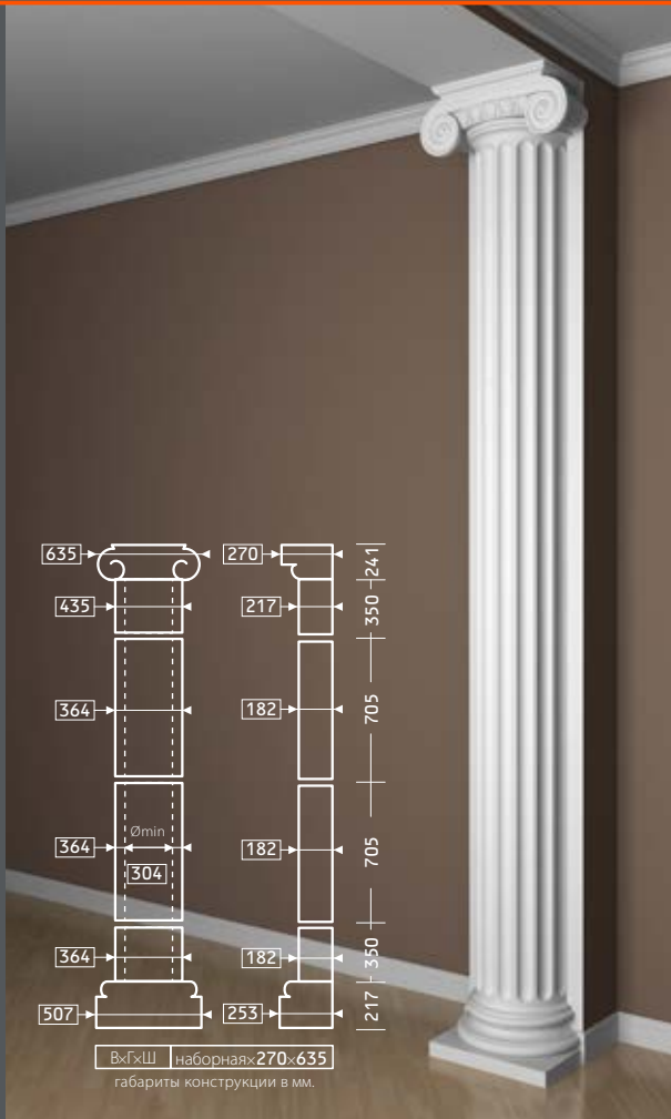
СТВОЛ 4.16.003
