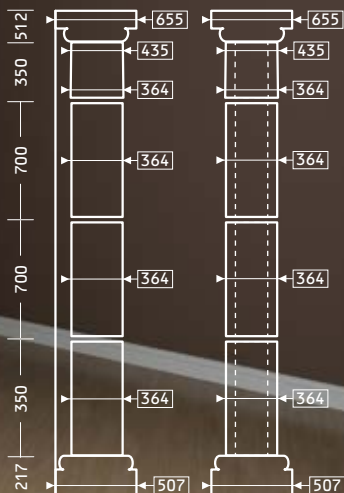
СТВОЛ 4.12.005
