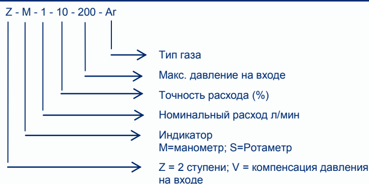
ОБОЗНАЧЕНИЕ ПО DIN EN 13918
