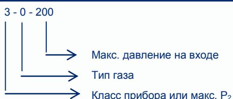
ОБОЗНАЧЕНИЕ ПО DIN EN ISO 2503
